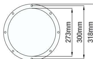
BOTTOM FLANGE
